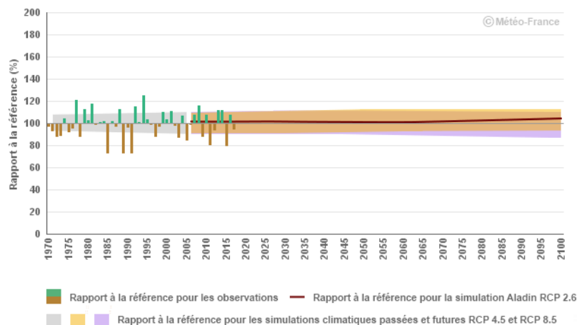
Figure 15 - Evolution des précipitations annuelles sur l'ancienne région Auvergne (Climat HD de Météo France)
