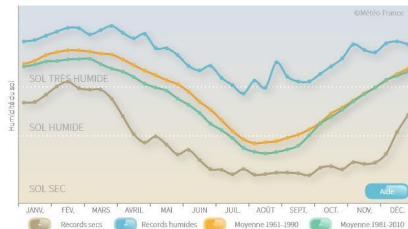
Figure 6 - Cycle annuel d'humidité du sol (moyenne et records) à Clermont-Ferrand (Climat HD de Météo France)
