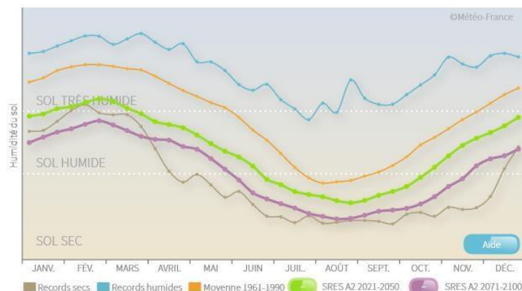
Figure 19 - Evolution du cycle annuel d'humidité en ancienne région Auvergne (Climat HD de Météo France)
