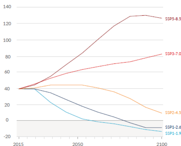
Figure 8 - Emissions de CO2 futures dans les cinq types d'évolution de la société (sixième rapport d'évolution du GIEC)
