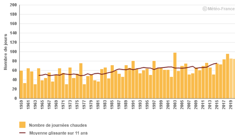
Figure 3 - Nombres de journées chaudes à Clermont-Ferrand sur la période 1959-2019 (Climat HD de Météo France)
