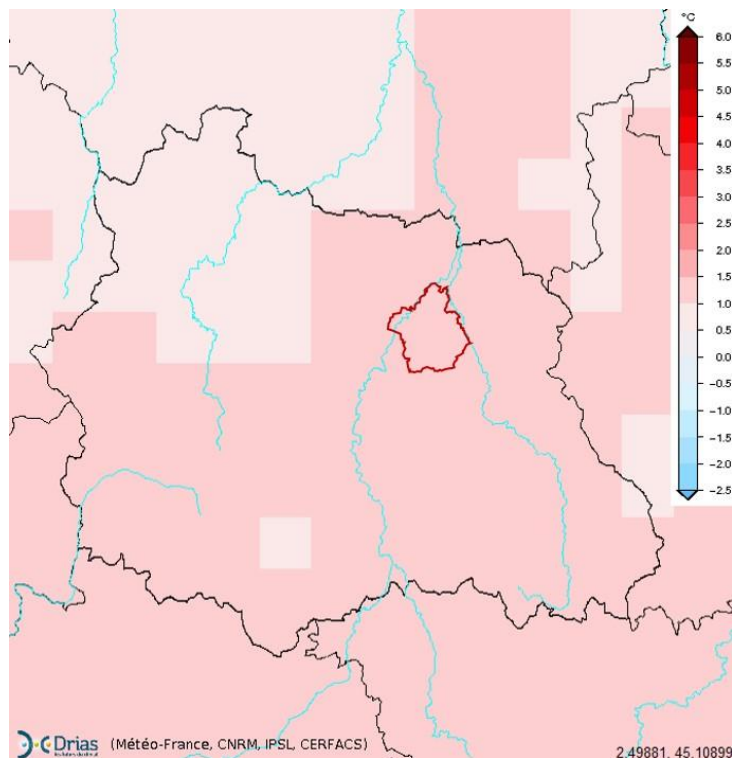
Figure 14 - Ecart de température moyenne [°C] : différence entre la période considérée et la période de référence sur un horizon proches (2021-2050) - RCP2.6 : Scénario avec politique climatique visant à faire baisser les concentrations en CO2 (DRIAS climat)
