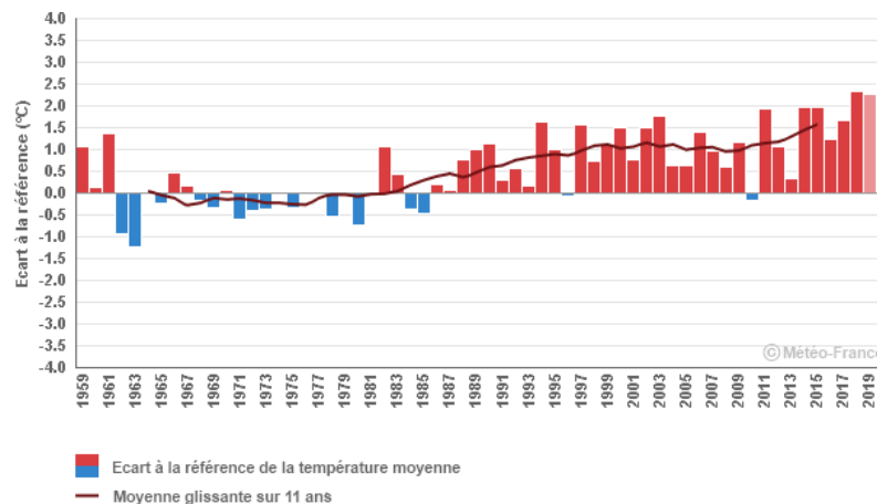
Figure 2 - Température moyenne annuelle : écart à la référence 1961-1990 à Clermont-Ferrand (Climat HD de Météo France)
