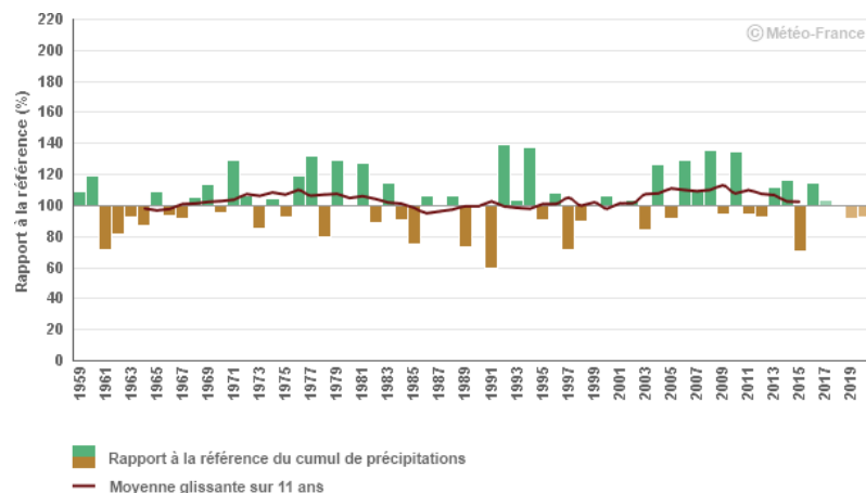
Figure 5 - Cumul annuel de précipitations : rapport à la référence 1961-1990 à Clermont-Ferrand (Climat HD de Météo France)
