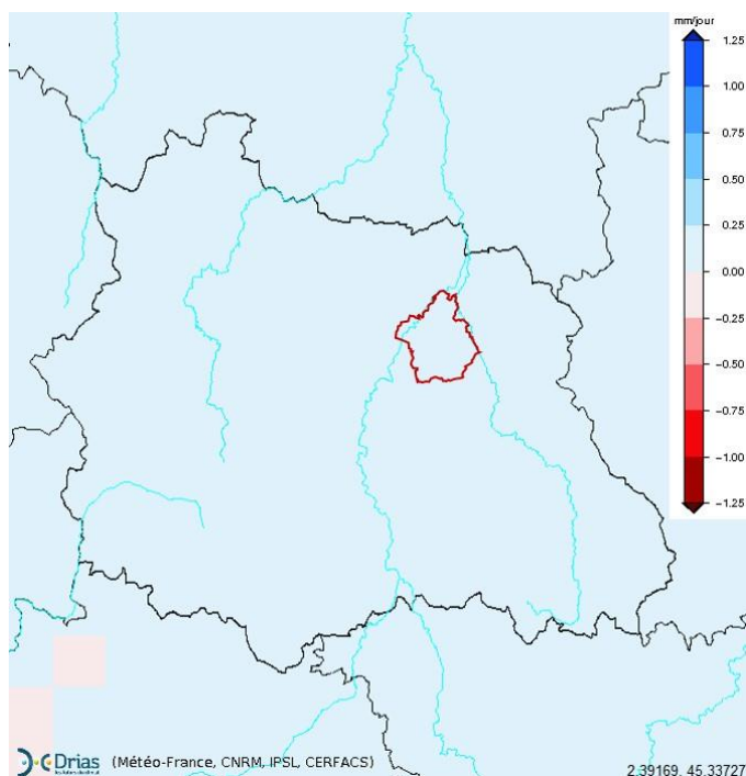
Figure 17 - Ecart de précipitations moyennes [mm] : différence entre la période considérée et la période de référence sur un horizon proches (2021-2050) - RCP8.5 : Scénario sans politique climatique (DRIAS climat)
