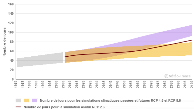
Figure 11 - Nombre de journées chaudes en Auvergne : simulations climatiques sur passé et futur pour trois scénarios
