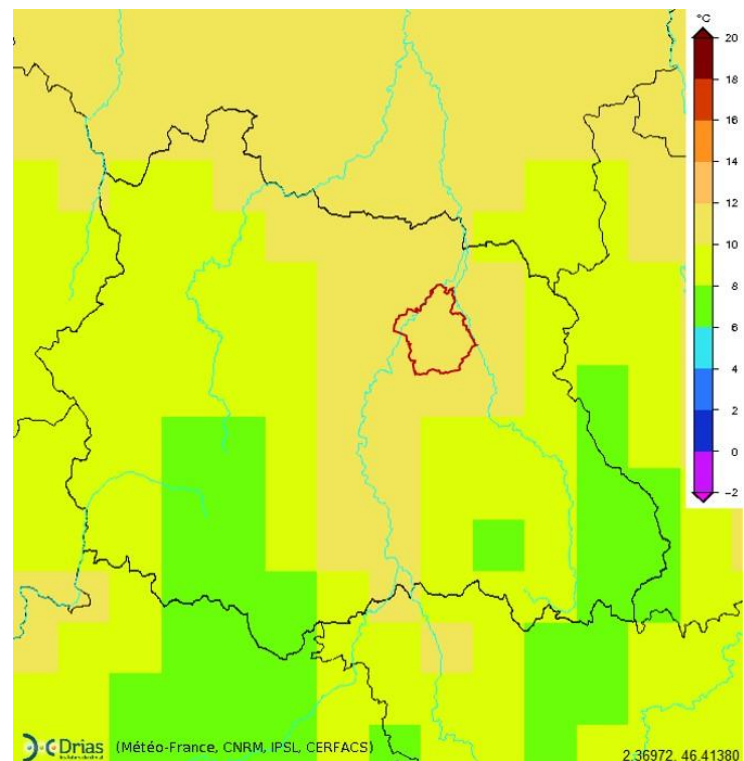
Figure 12 - Température moyenne annuelle (°C) - données de référence actuelle (DRIAS climat)
