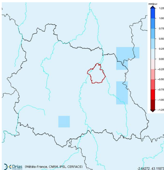
Figure 18 - Ecart de précipitations moyennes [mm] : différence entre la période considérée et la période de référence sur un horizon proches (2021-2050) - RCP2.6 : Scénario avec une politique climatique visant à faire baisser les concentrations en CO2 (DRIAS climat)
