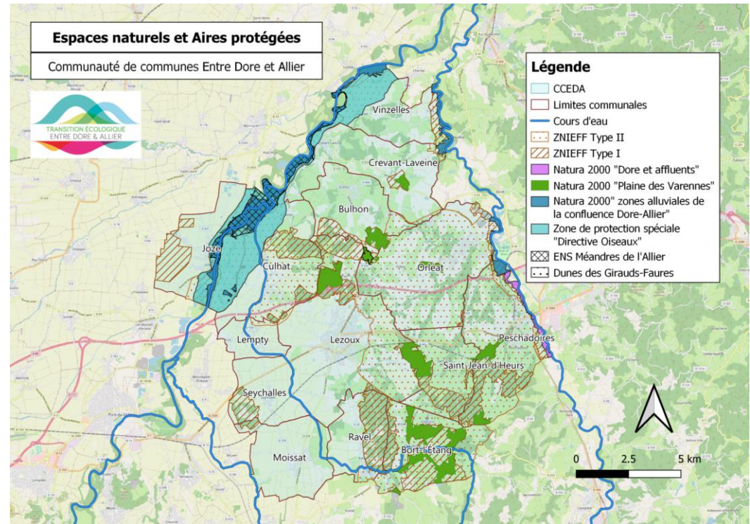
Figure 23 - Espaces naturels à enjeux de préservation, incluant zones Natura 2000 et Directives spécifiques, sur le territoire de la CCEDA
