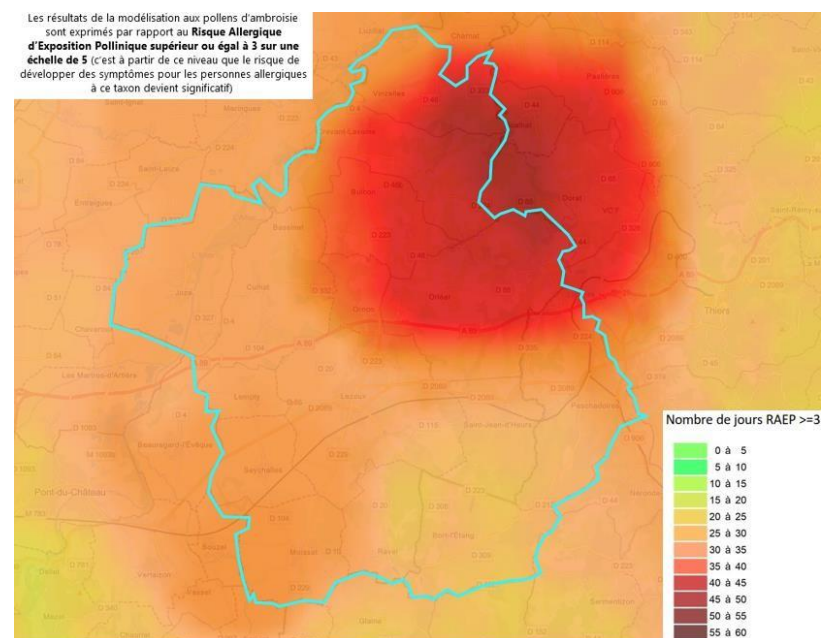
Figure 30 - Estimation du risque allergique lié à l'ambrosie sur la CCEDA en 2020 (Vizea d'après ATMO AURA)
