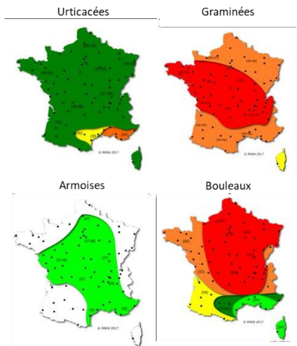
Figure 31 - Risques allergiques pour les urticacées, graminées, armoises et bouleaux (RNSA, 2017)
