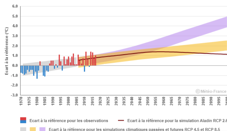
Figure 10 - Evolution de la température moyenne annuelle en ancienne région Auvergne (Climat HD de Météo France)
