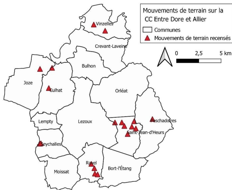
Figure 26 - mouvements de terrain recensés sur le territoire de la CCEDA (Vizea)
