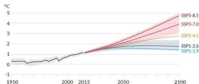
Figure 1 - Evolution des températures selon les différents scénarios (SSP) - 14CE
