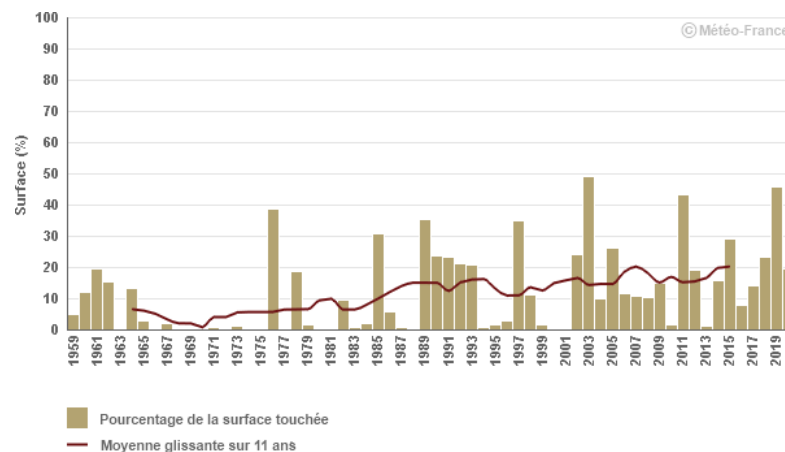
Figure 4 - Pourcentage de la surface touchée sur la période 1959-2019 (Climat HD de Météo France)
