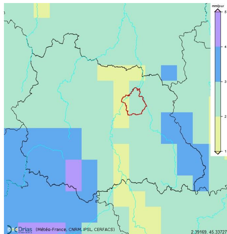
Figure 16 - Précipitations moyennes (mm) - données de référence actuelles (DRIAS climat)
