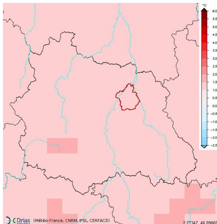
Figure 13 - Ecart de température moyenne [°C] : différence entre la période considérée et la période de référence sur un horizon proches (2021-2050) - RCP8.5 : Scénario sans politique climatique (DRIAS climat)
