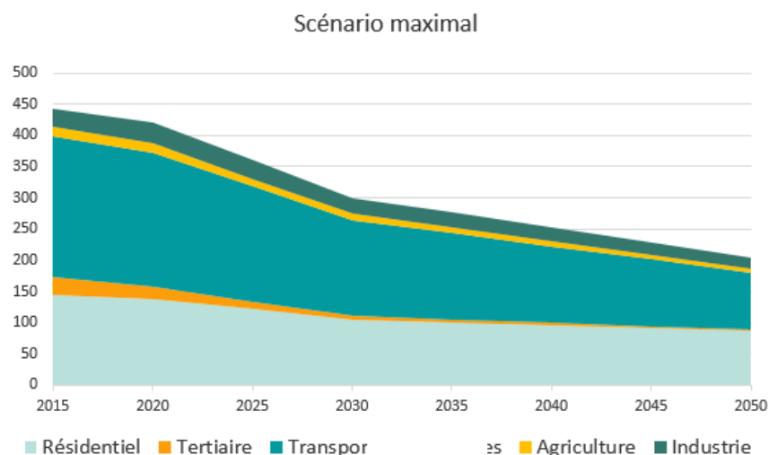
Figure 10 - Evolution des consommations d'énergie finale (en GWh/an) à l'horizon 2050 de la CC Entre Dore et Allier selon le scénario maximal - Vizea, 2022
