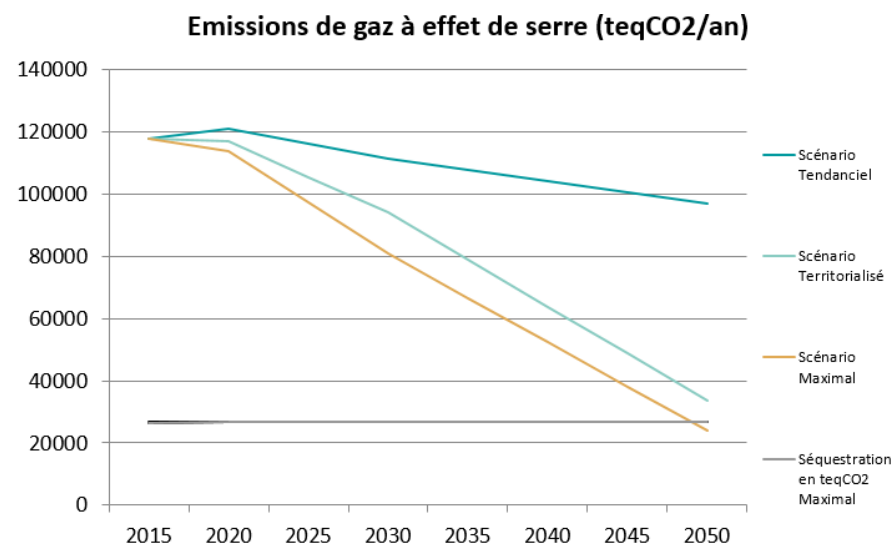
Figure 18 – Evolution des émissions de GES de la CC Entre Dore et Allier en teqCO 2 /an, Vizea, 2022
